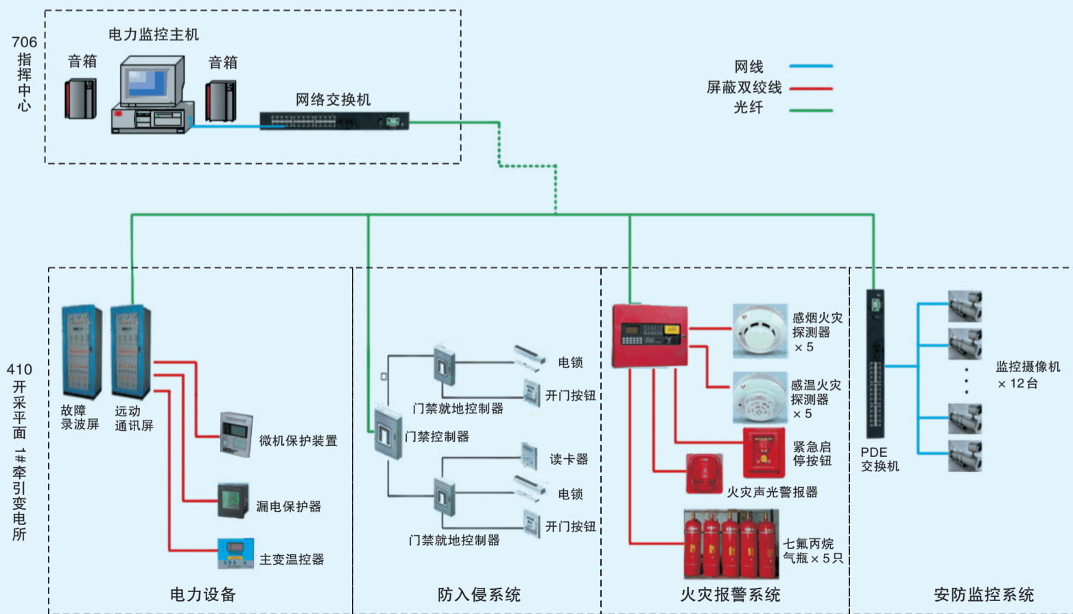
北方铜业铜峪矿1#牵引变电所无人值守系统
